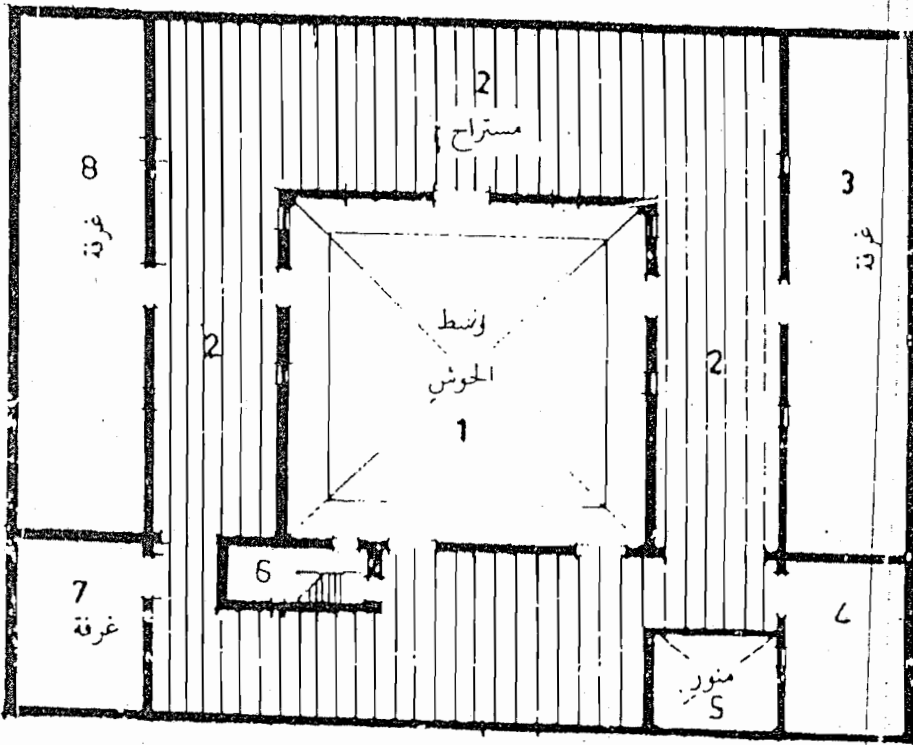
مسقط افقي للبيت الطرابلسي
